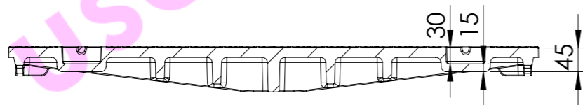
COUPE A-A
