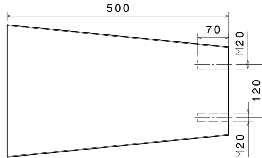
Vue de gauche Echelle : 1:5
