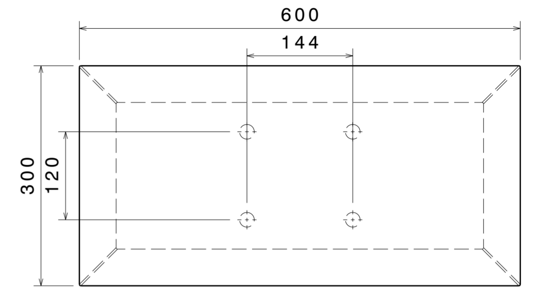
Vue de derriere Echelle : 1:5
