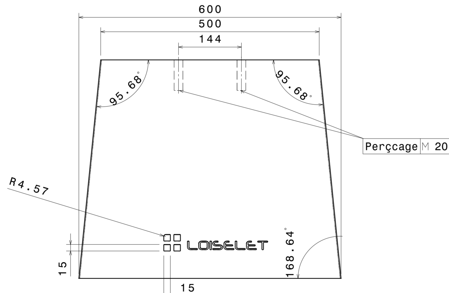
Vue de dessous Echelle : 1:5
